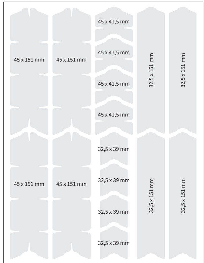
Hinterbau
