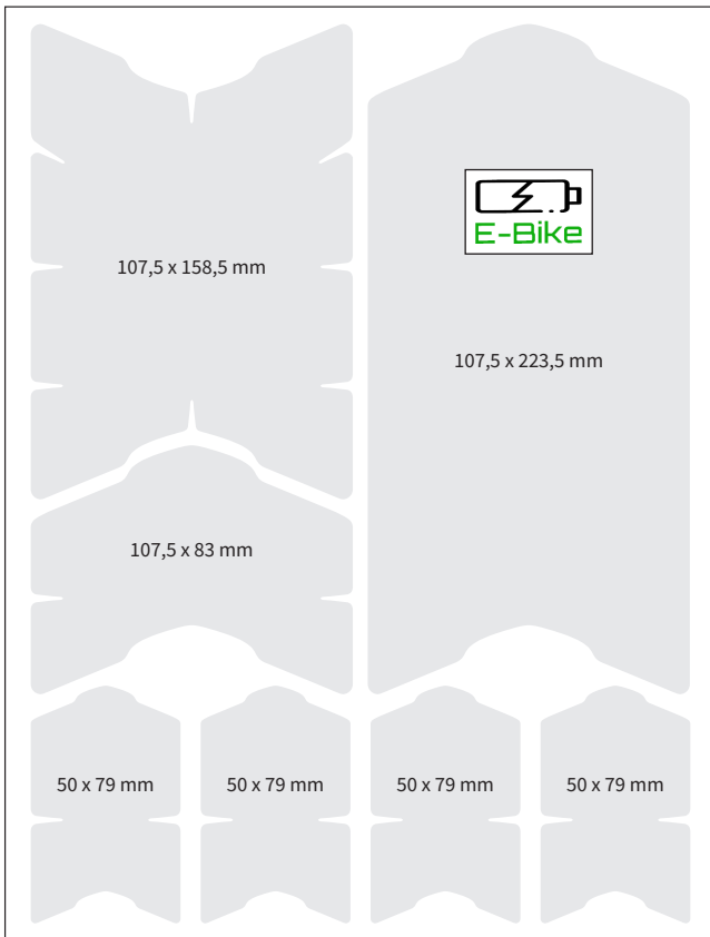
Unterrohr + Sitzrohr E-Bike
