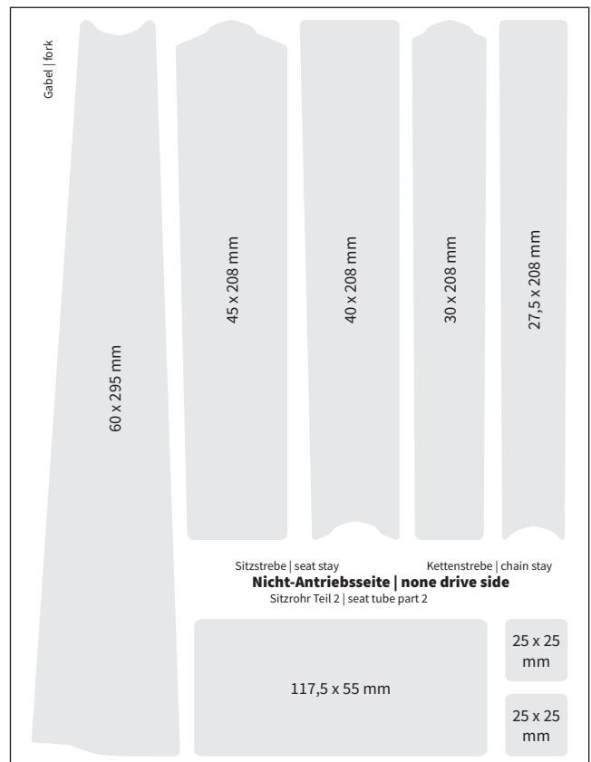
Sitzrohr, Sitz- und Kettenstrebe, Gabel Nichtantriebsseite
