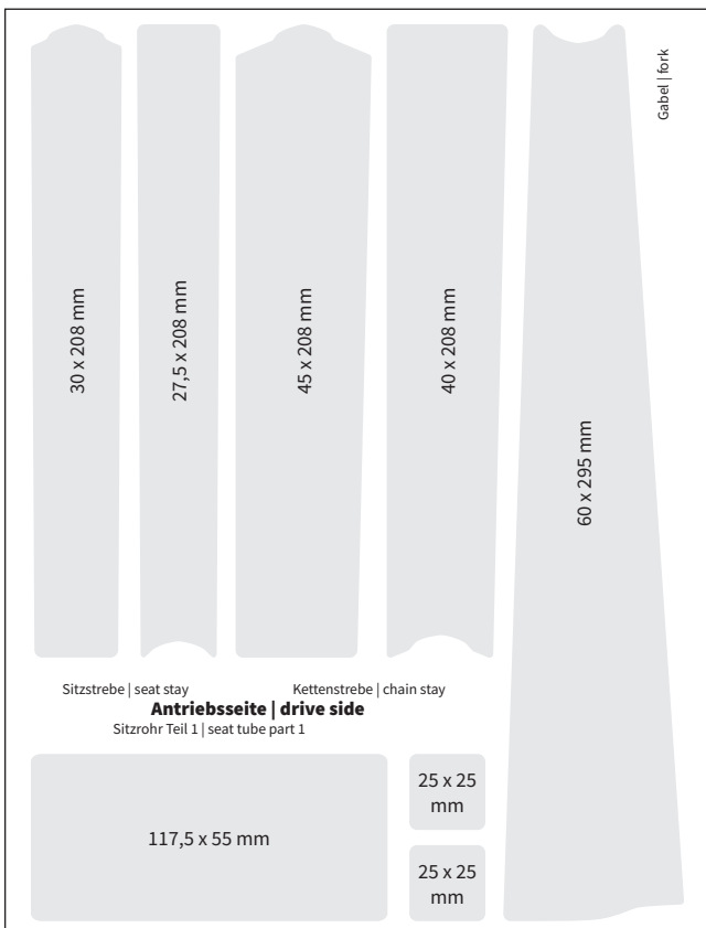
Sitzrohr, Sitz- und Kettenstrebe, Gabel Antriebsseite
